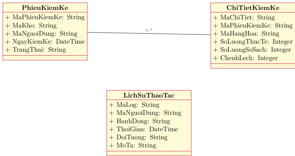
Figure 1: Sơ đồ lớp kiểm kê và lịch sử thao tác
